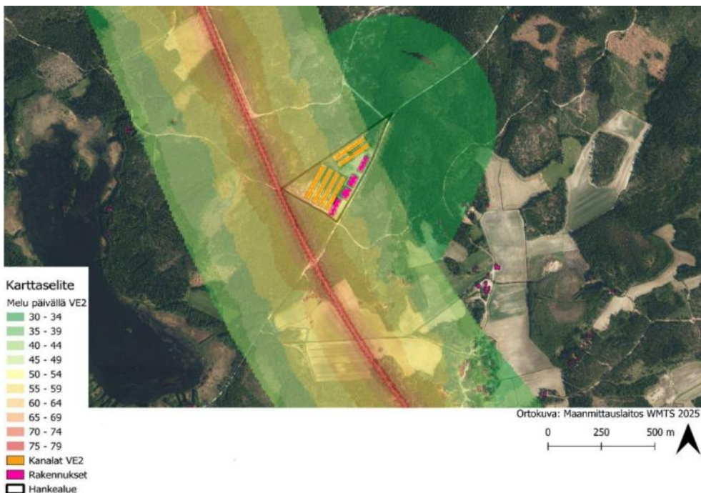
Kuva 6. Liikenteen aiheuttama melu päiväaikaan, VE2 (6 kanala). Lähde: Munituskanalan melumallinnus (Fertilex Oy), kuva 9. Macon Oy.
