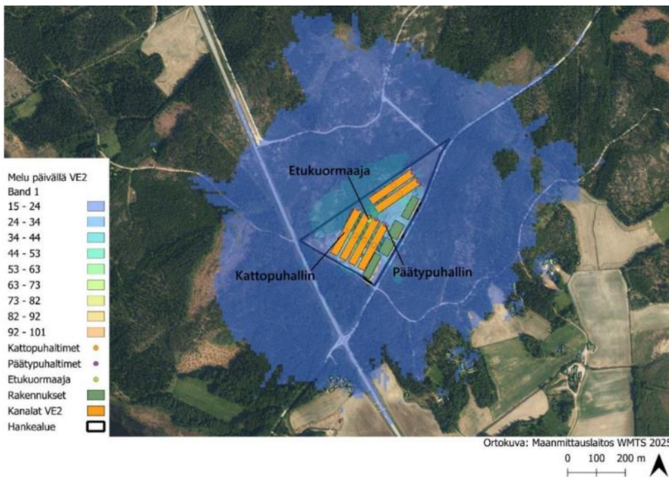
Kuva 10. Kanalan aiheuttama melu päiväaikaan, VE2 (6 kanalia). Lähde: Munituskanalan melumallinnus (Fertilex Oy), kuva 18. Macon Oy.
