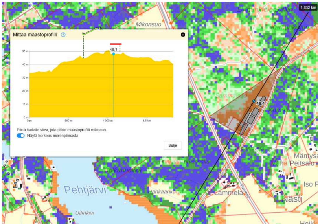
Kuva 17. Maaston leikkausprofiili ja leikkauslinjan sijainti kartalla. Katselusuunta luoteeseen. Leikkausprofiililla oleva punainen viiva sijaitsee noin korkeudessa +56 m, joka vastaa suunnilleen nykyisten ja tulevien kanalarakennusten harjakorkeutta. Vihreä katkoviiva profiilikuvan yläreunassa, osittain ulkopuolella, vastaa suunnilleen 18 m korkeaa puustoa valtatie ja kanalan välisellä alueella. Lähde: Paikkatietoikkuna, josta MML:n "Taustakartta", "Peruskarttarasterin rakennukset" ja "Kiinteistöjaotus" sekä Luonnonvarakeskuksen "Puuston keskipituus 2023 (dm)".
